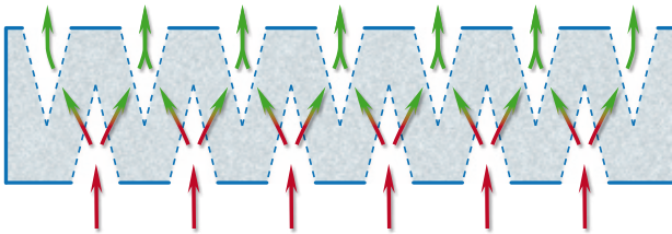
CarbonMax filter Prinzip
